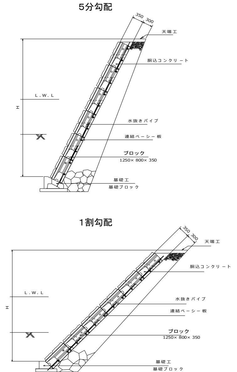
標準断面図
