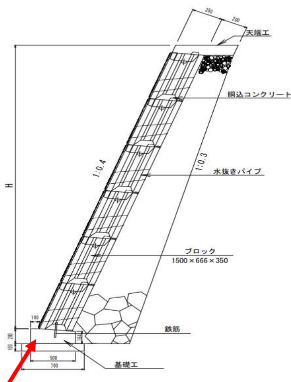
<4分断面図>
