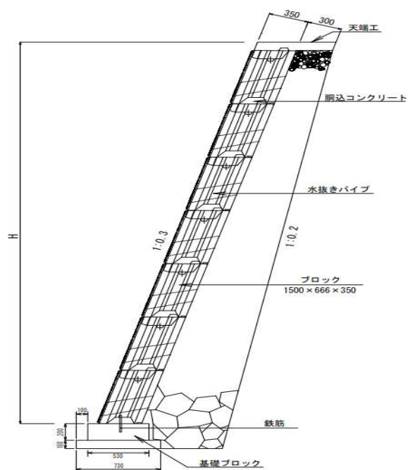
<3分断面図>
