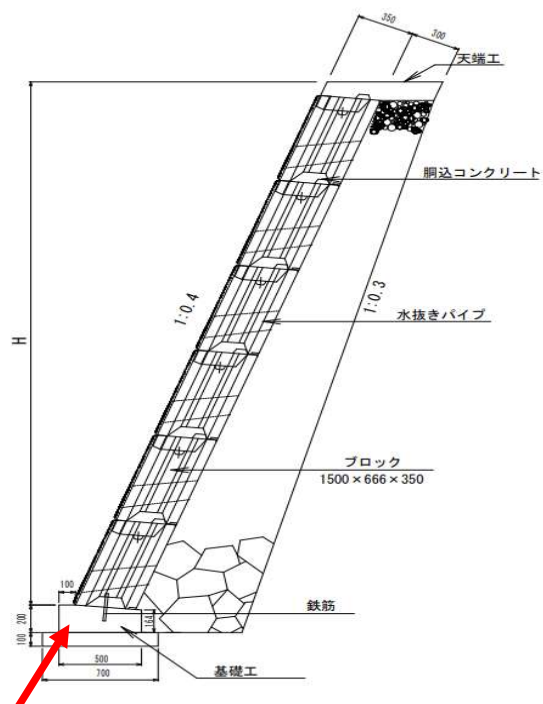
<4分断面図>
