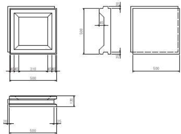
張りブロック 500×500×120
