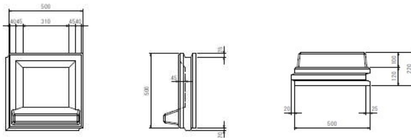
張りブロック120mm 防災用
